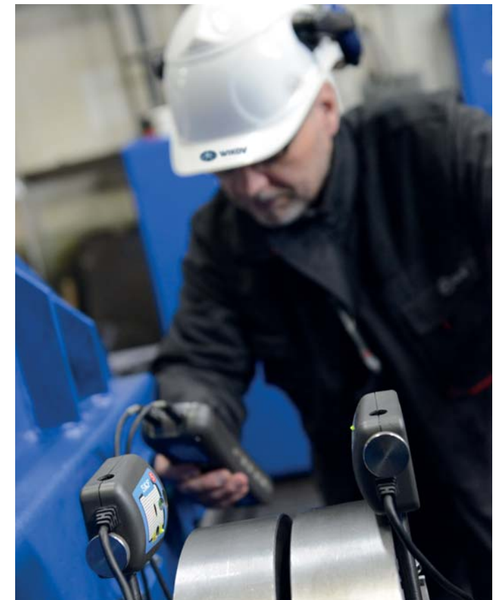
osové vyrovnání hřídelí
